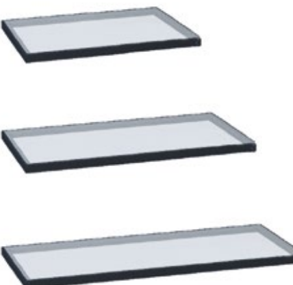
Ripiano metallo e vetro 1438T/120, L. 120 H. 3,5 P. 47,3 1438T/90, L. 90 H. 3,5 P. 47,3 1438T/60, L. 60 H. 3,5 P. 47,3
